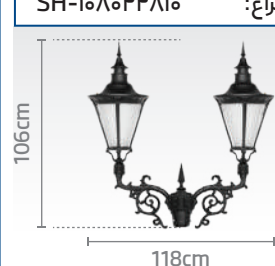
کد چراغ: SH-۱۰۸۰۲۲۱۰۱۰
